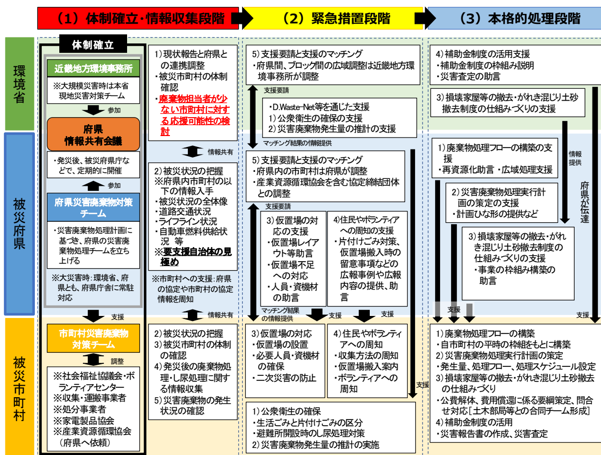
図 県を核にした災害廃棄物処理対策の行動フロー図例
