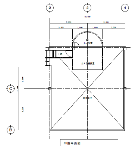
PH階平面図
