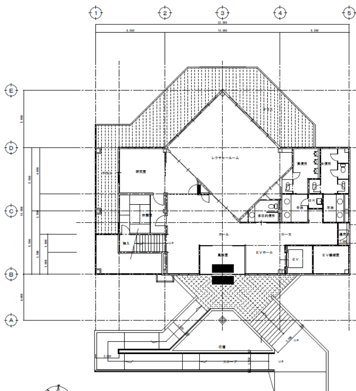
1階平面図
