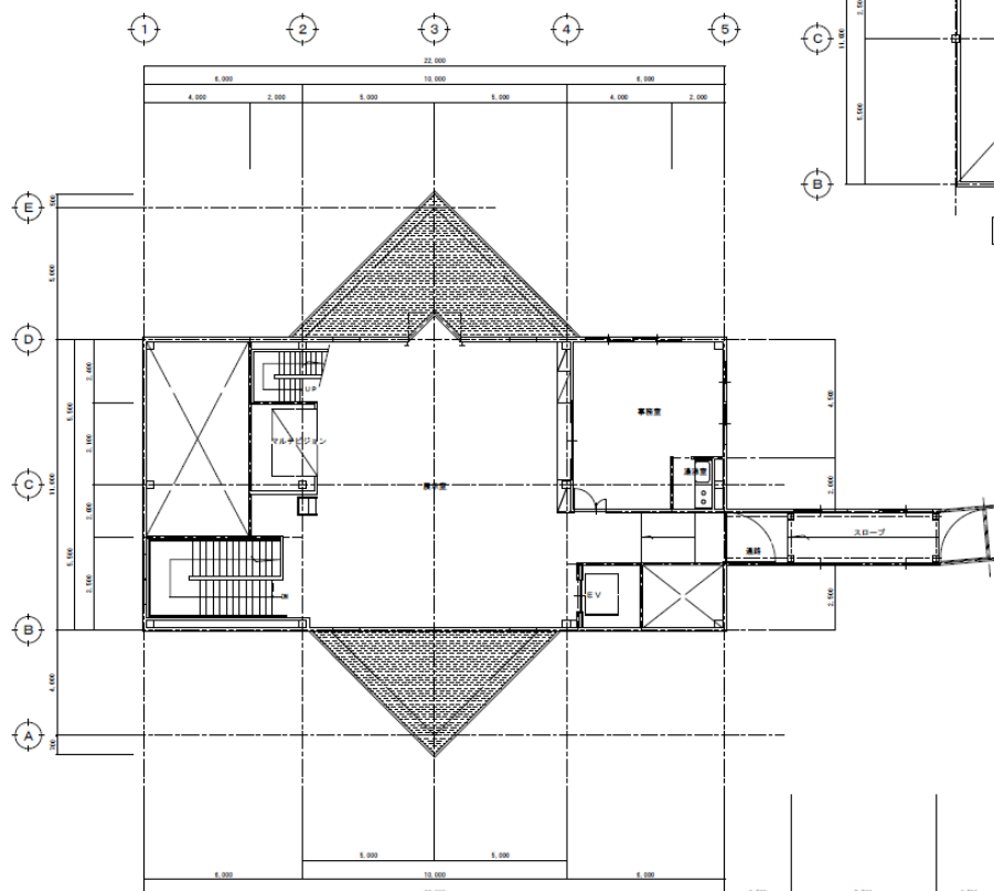
2階平面図
