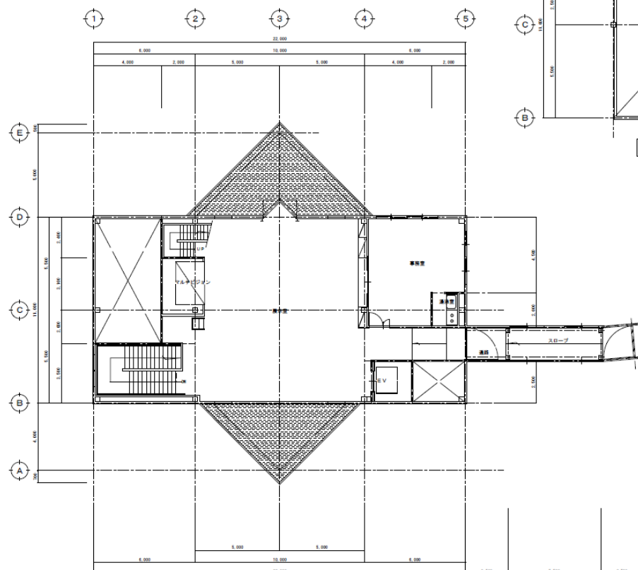
2階平面図
