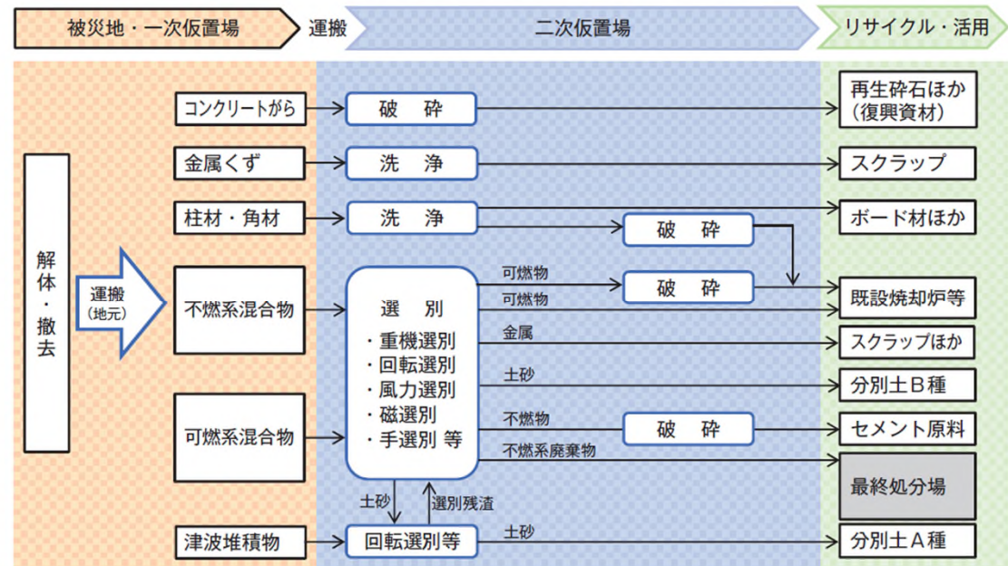
図 3.5.2 標準的な処理の流れ
