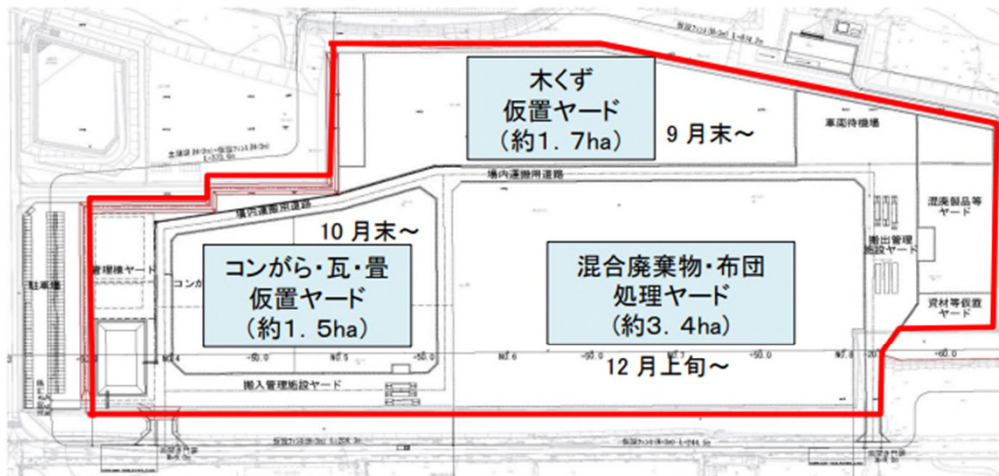
図3-8 二次仮置場平面図
