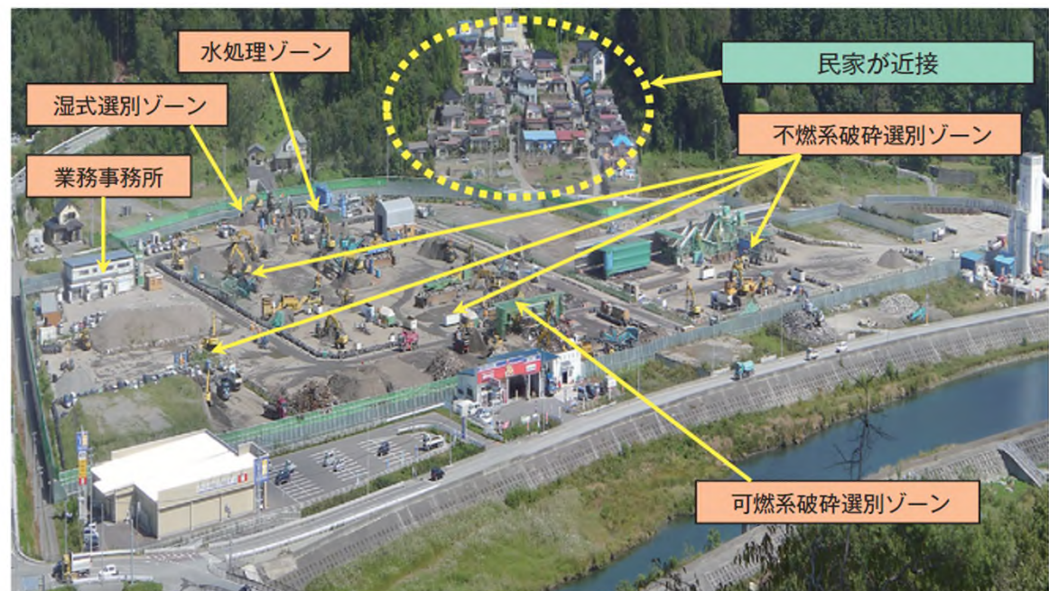
写真 3.5.10 二次仮置場の施設配置状況
