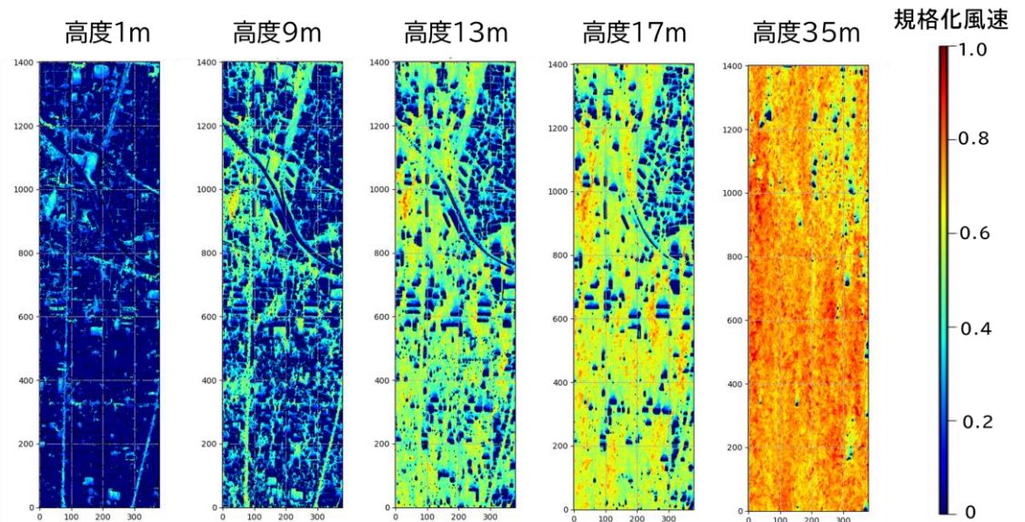
様々な高度で評価された風速の空間分布
