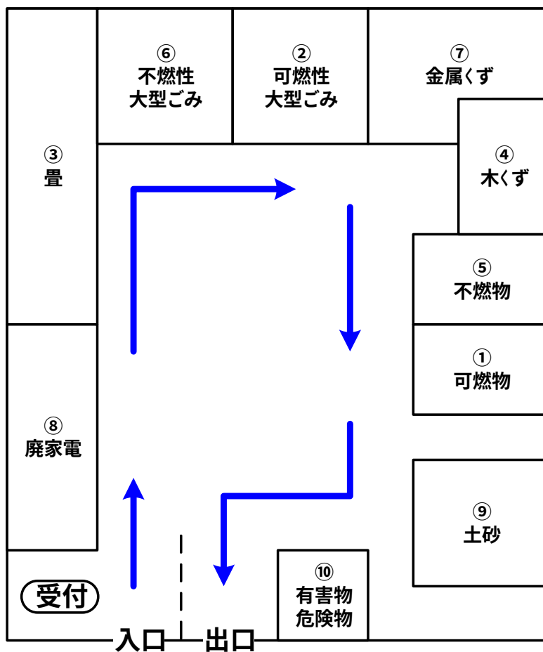
図 3-2 仮置場レイアウト例
