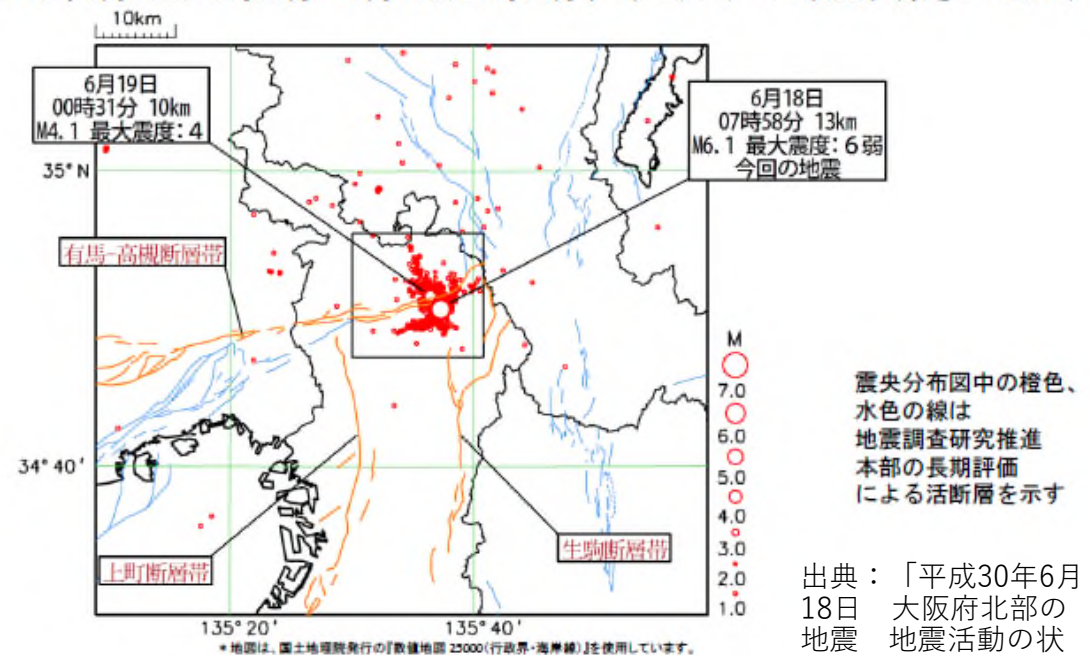
震央分布図 (2018年6月18日00時00分～8月17日09時00分、マグニチュード * 1.0以上、深さ0～20km)
