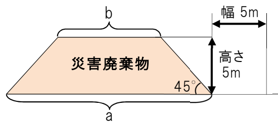
横断面図
