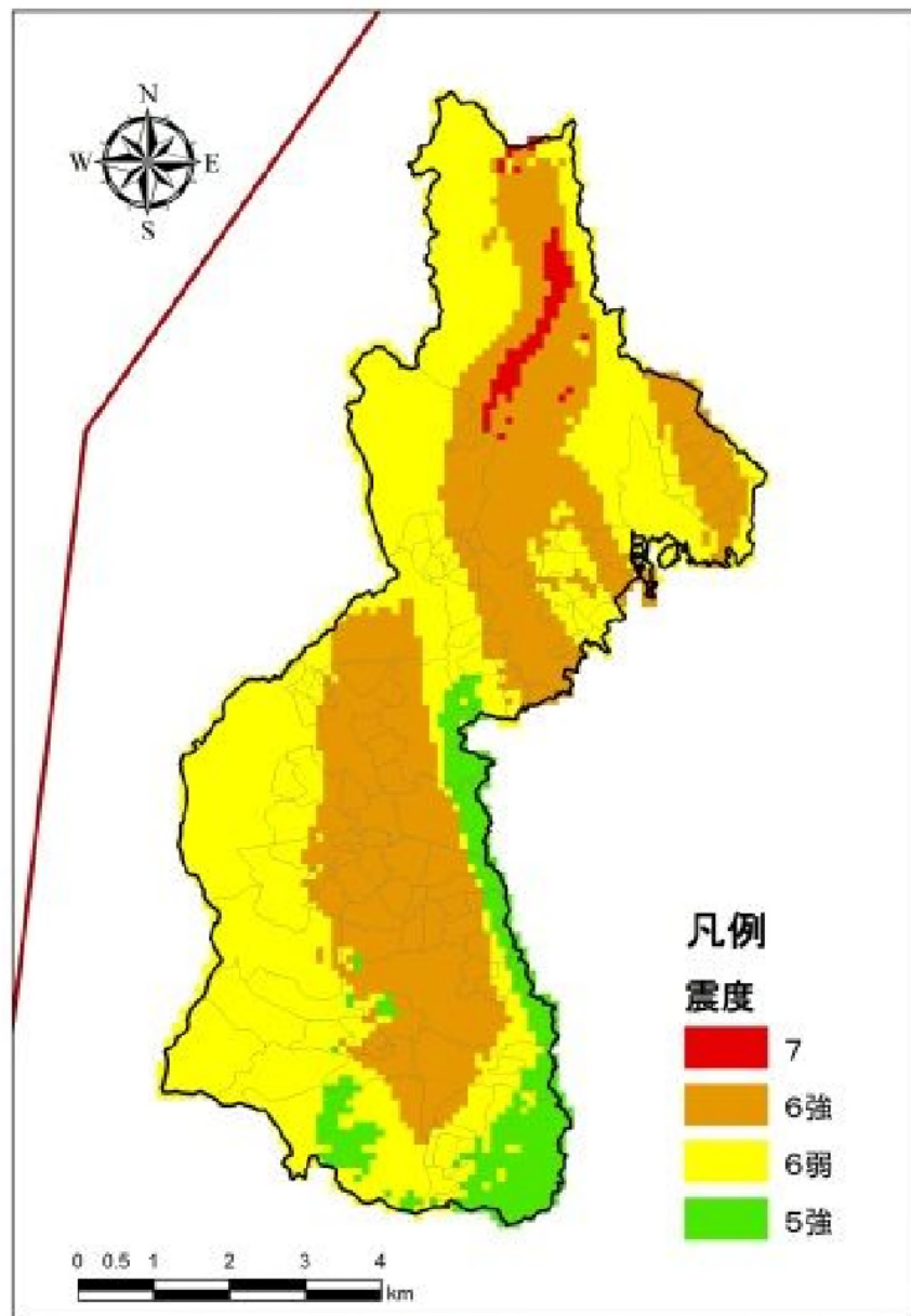
図 1.2.1 生駒断層帯震度分布図
