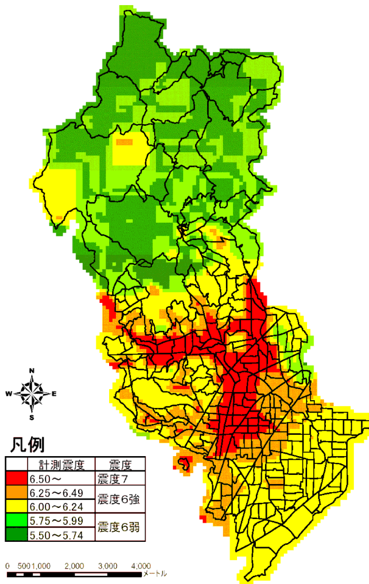
図 1.2.1 有馬高槻断層帯地震 震度分布図
