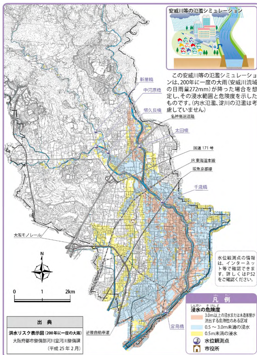
図 1.3.1 安威川等の氾濫シミュレーション
