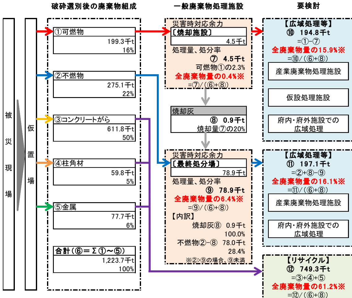
図 3.2.3 生駒断層帯地震の災害廃棄物処理フロー
