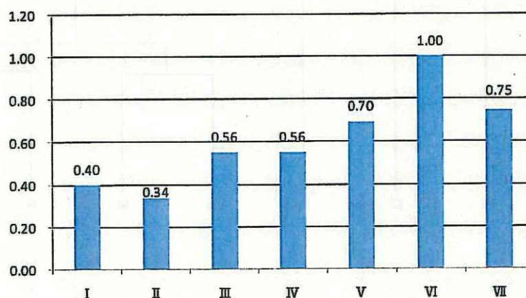
図 5-21 食材性昆虫類の補正(※)した多様度指数 (H17-18 年：柵内外合計累積) (※個体数の多い Sepedophilus sp. と Epuraea spp. を 1 個体として補正して計算した)
