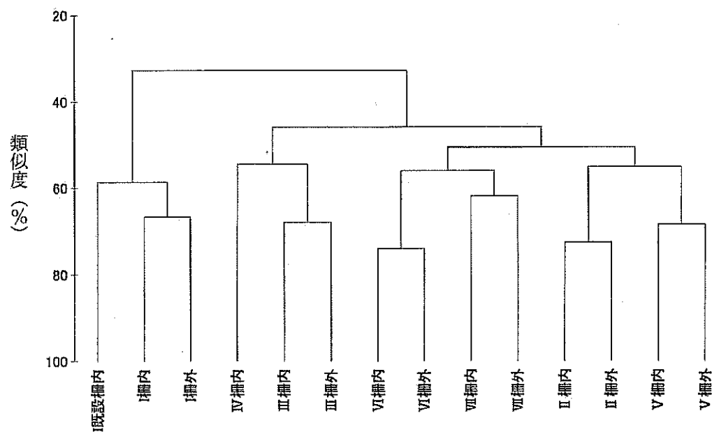
図 5-12 各植生タイプにおける土壌動物群集の類似度 (Bray-Curtis 指数) に基づく樹形図
