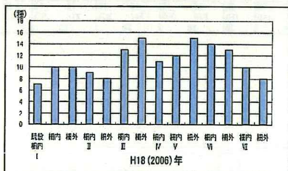
図 5-7 各植生タイプにおける 年ごとの地表性甲虫の種数
