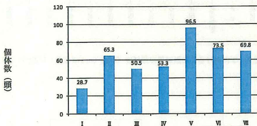
図 5-26 各植生タイプにおけるクモ類の個体数 (H16-H18 年：柵内外合計累積)
