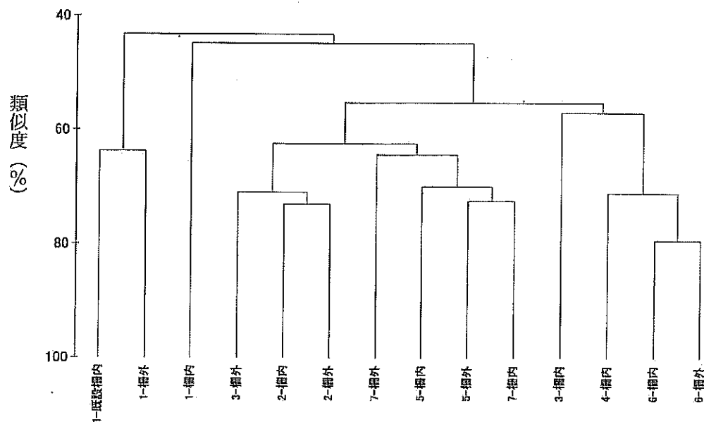
図 5-4 各植生タイプにおける地表性甲虫群集の類似度 (Bray-Curtis 指数) に基づく樹形図
