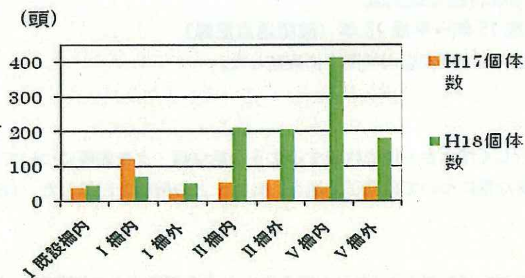
図 5-30 ミヤコザサ林床の各植生タイプにおける草本層のクモ個体数
