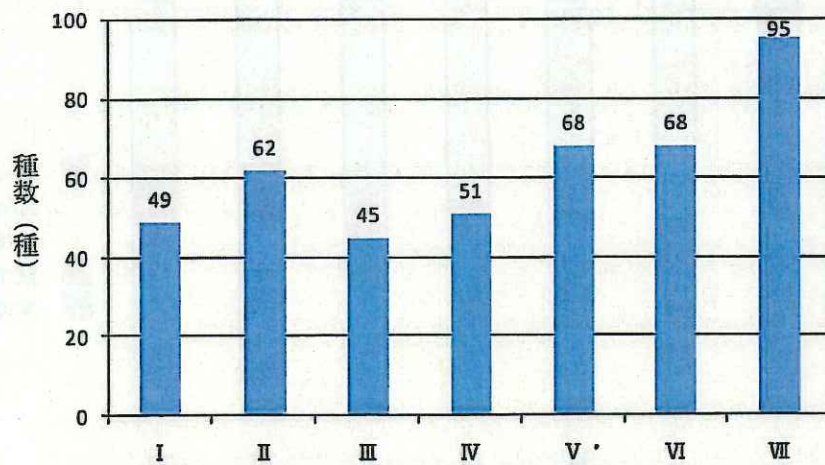
図 5-14 各植生タイプにおけるガ類の種数
