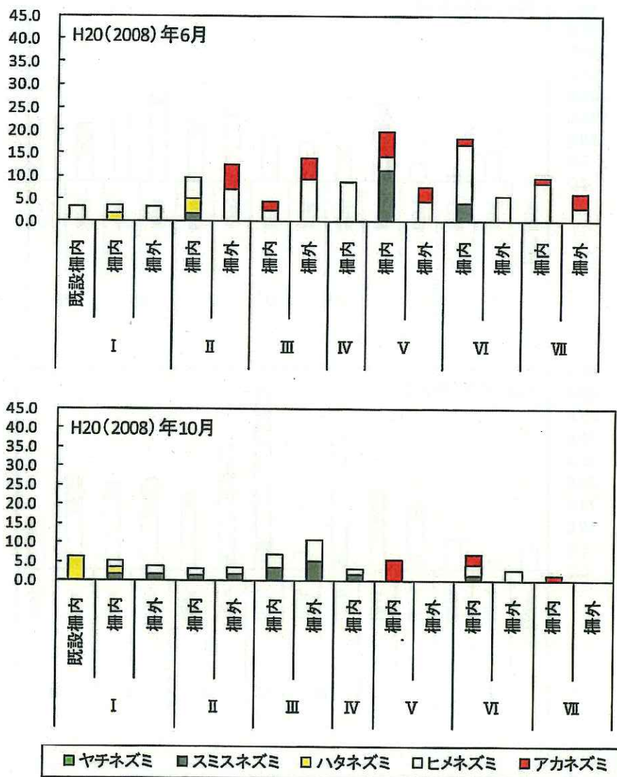
図 1-2 各植生タイプにおいてシャーマントラップにて確認されたネズミ類 (H20 年)
