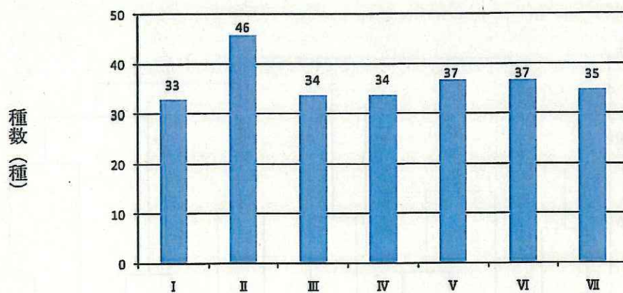
図 5-25 各植生タイプにおけるクモ類の種数 (H16-H18 年) (柵内外合計累積：1 対照区当たり年間)
