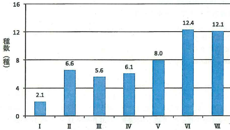
図 5-9 大型土壌動物の種数 (H17-H18 年：柵内外合計累積)
