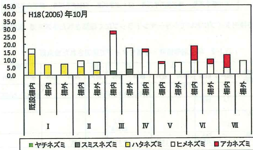
図 1-1 各植生タイプにおいてシャーマントラップにて確認されたネズミ類 (H16 年と H18 年)
