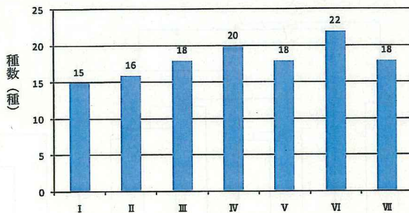
図 5-1 地表性甲虫類の種数 (H16-H18 年：柵内外合計累積)
