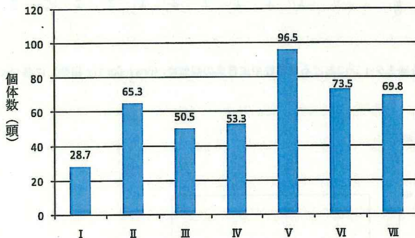
図 5-2 地表性甲虫類の個体数 (H16-H18 年：柵内外合計累積：1 対照区当たり年間)
