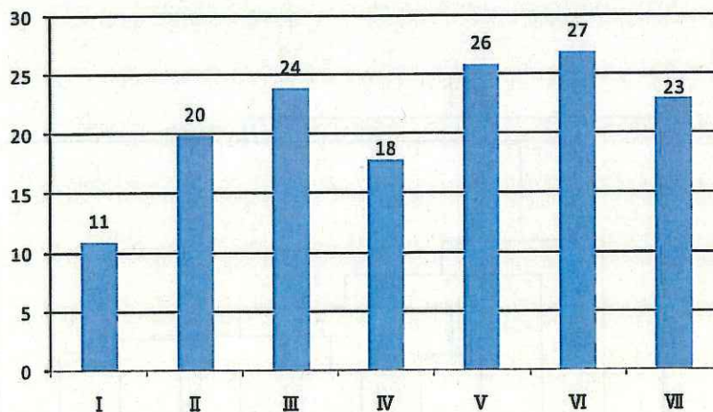
図 5-19 食材性昆虫類の種数 (H17-H18 年：柵内外合計累積)
