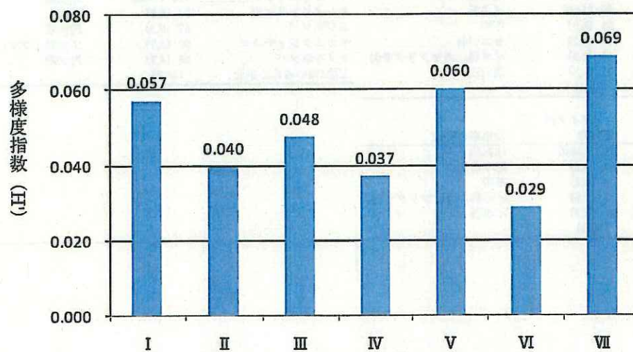
図 5-16 各植生タイプにおけるガ類の多様度指数 ( H' )
