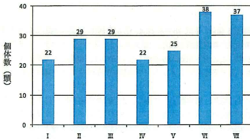
図 5-10 大型土壌動物の個体数 (H17-H18 年：柵内外合計累積：1 対照区当たり年間)
