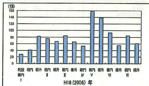
図 5-8 各植生タイプにおける 年ごとの地表性甲虫の個体数
