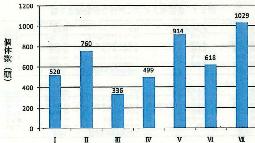
図 5-15 各植生タイプにおけるガ類の個体数
