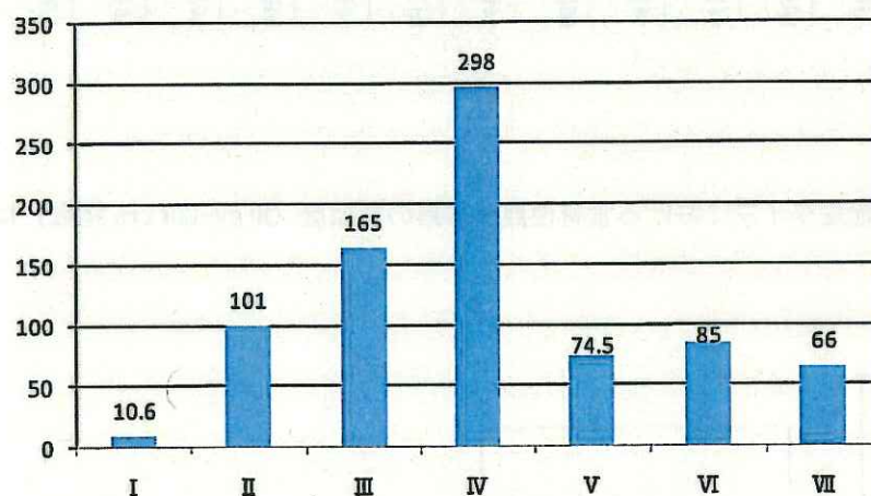
図 5-20 食材性昆虫類の個体数 (H17-18 年：柵内外合計累積：1 対照区当たり年間)
