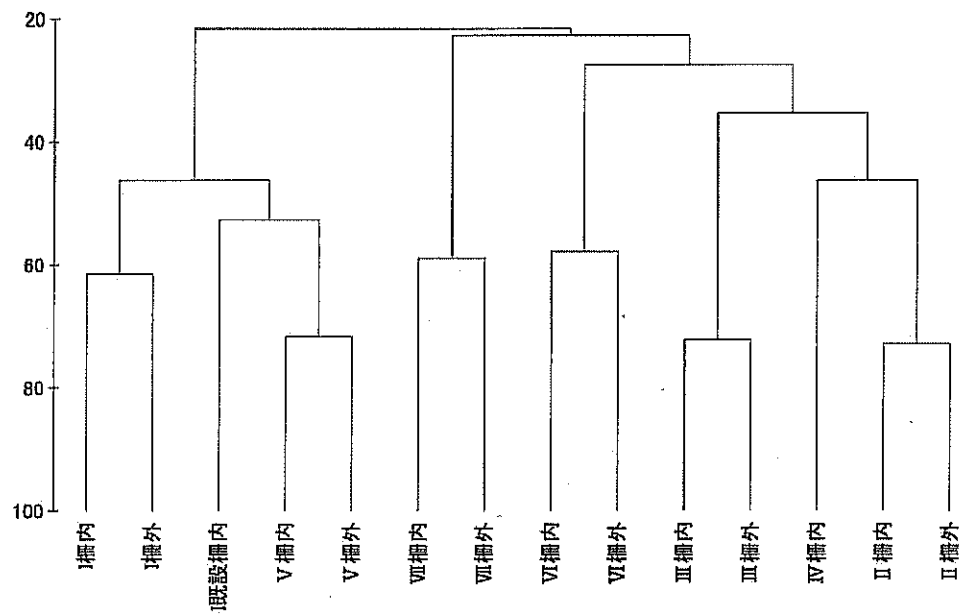
図 5-28 各植生タイプにおけるクモ類群集の類似度 (Bray-Curtis 指数) に基づく樹形図
