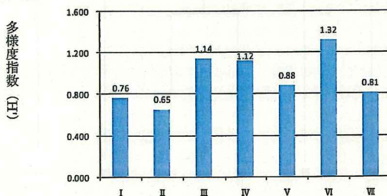
図 5-27 各植生タイプにおけるクモ類の多様度指数 (H16-H18 年：柵内外合計累積)
