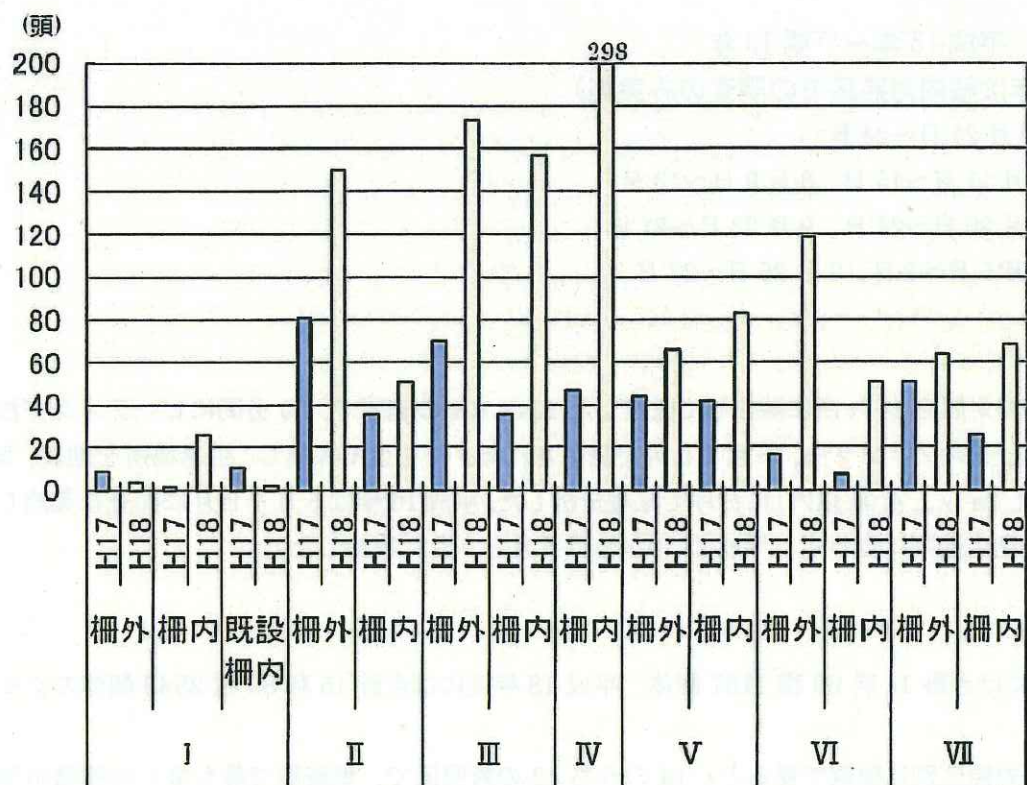
図 5-24 各植生タイプにおける食材性昆虫類の個体数 (各年・柵内外別)
