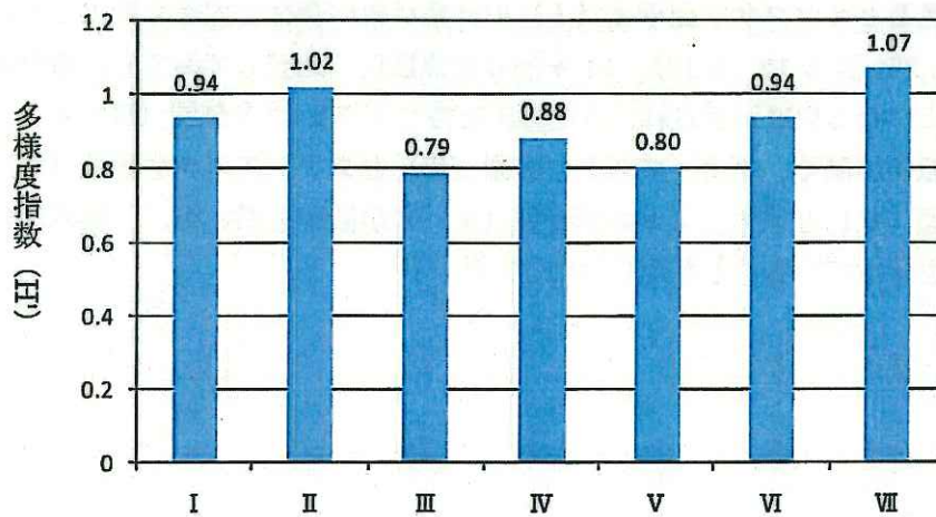
図 5-11 大型土壌動物の多様度指数 (H') (H16-H18 年：柵内外合計累積)
