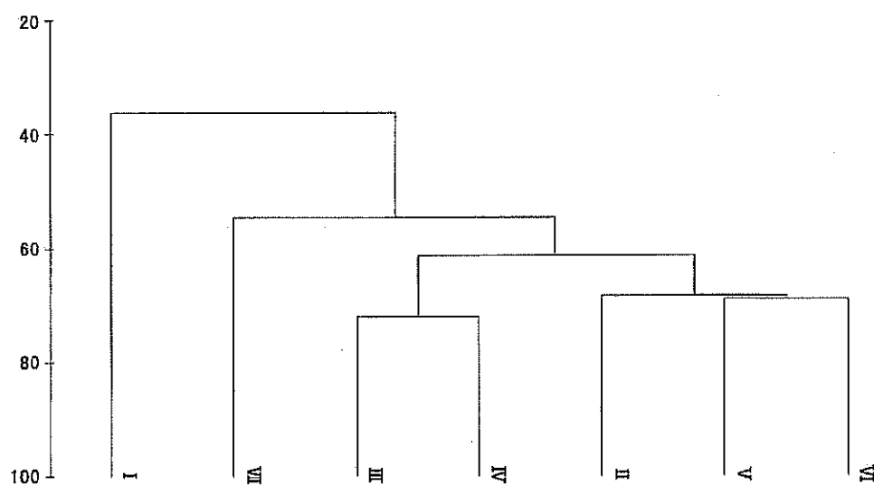
図 5-18 各植生タイプにおけるガ類群集の類似度 (Bray-Curtis 指数) に基づく樹形図
