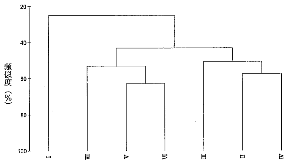
図 5-13 各植生タイプにおける土壌動物群集の類似度 (Bray-Curtis 指数) に基づく樹形図 (柵内・柵外統合)
