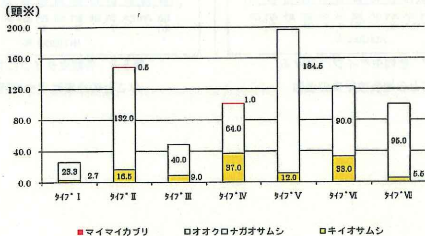
図 5-6 植生タイプ別のオサムシ類の出現状況 (H16-18 年累計) (※1 対象区あたり年間合計個体数に変換)
