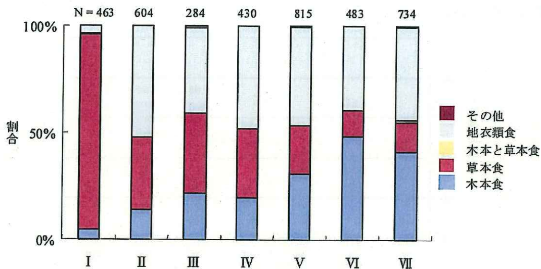
図 5-17 各植生タイプにおける出現種の幼虫期の植生の割合 (個体数)
