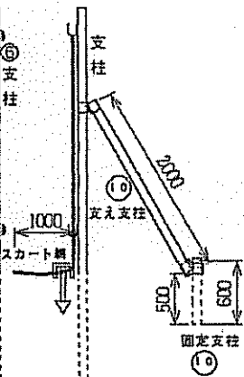
設置側面図
