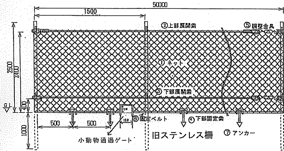
設置側面図
