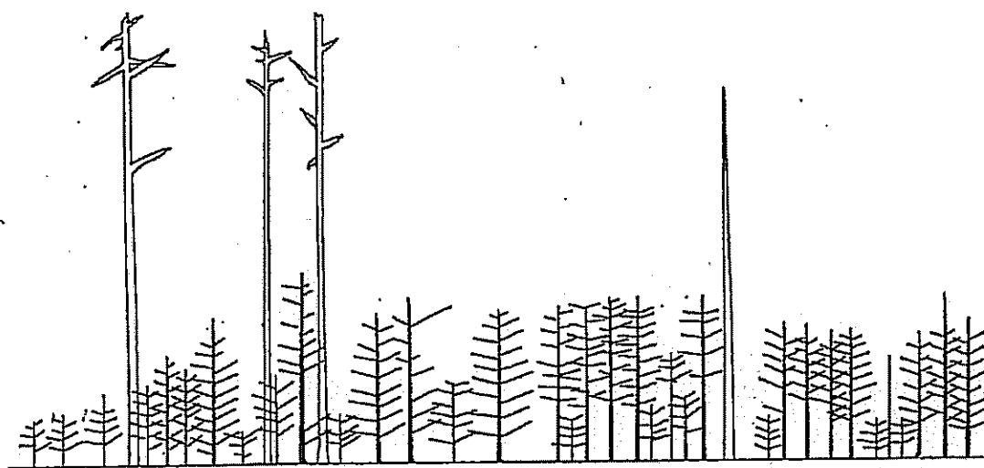
図3 正木峠~正木原 トウヒ林再生林断面図 (白は枯死木、Cはヒノキ)
