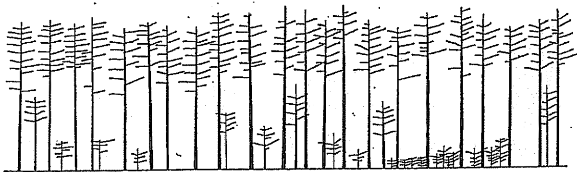
図1 正木峠~正木原 トウヒ林壮令林断面図
