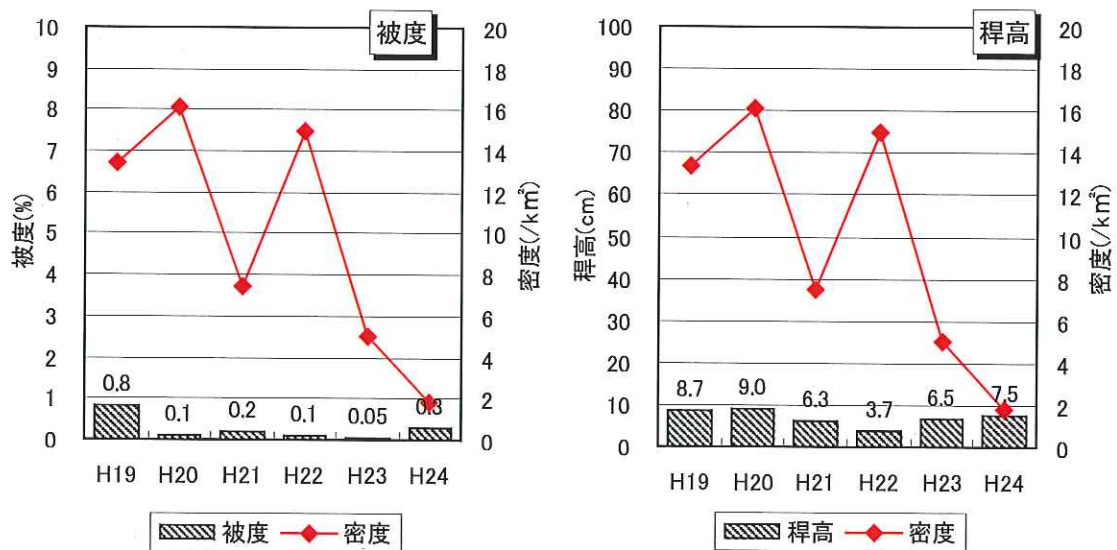
図19 平成19～24年度のスズタケの被度と稈高の変化とニホンジカの生息密度の変化 (重点監視地区N7)
