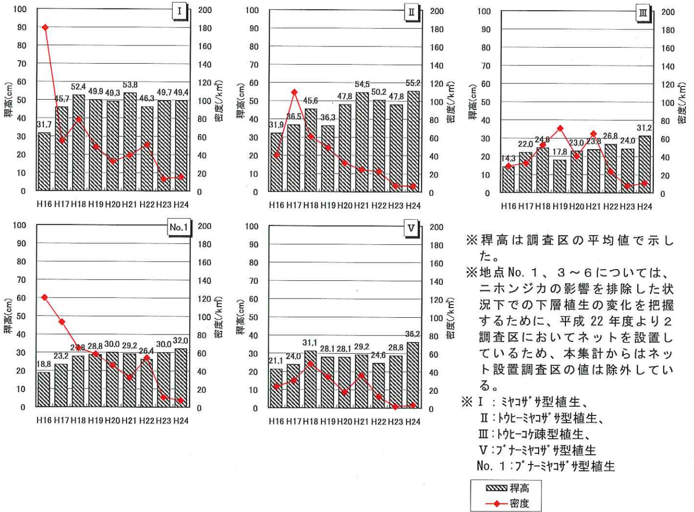
図 20(1) ササ型植生における平成 16～24 年度のミヤコザサの稈高とニホンジカ生息密度の変化
