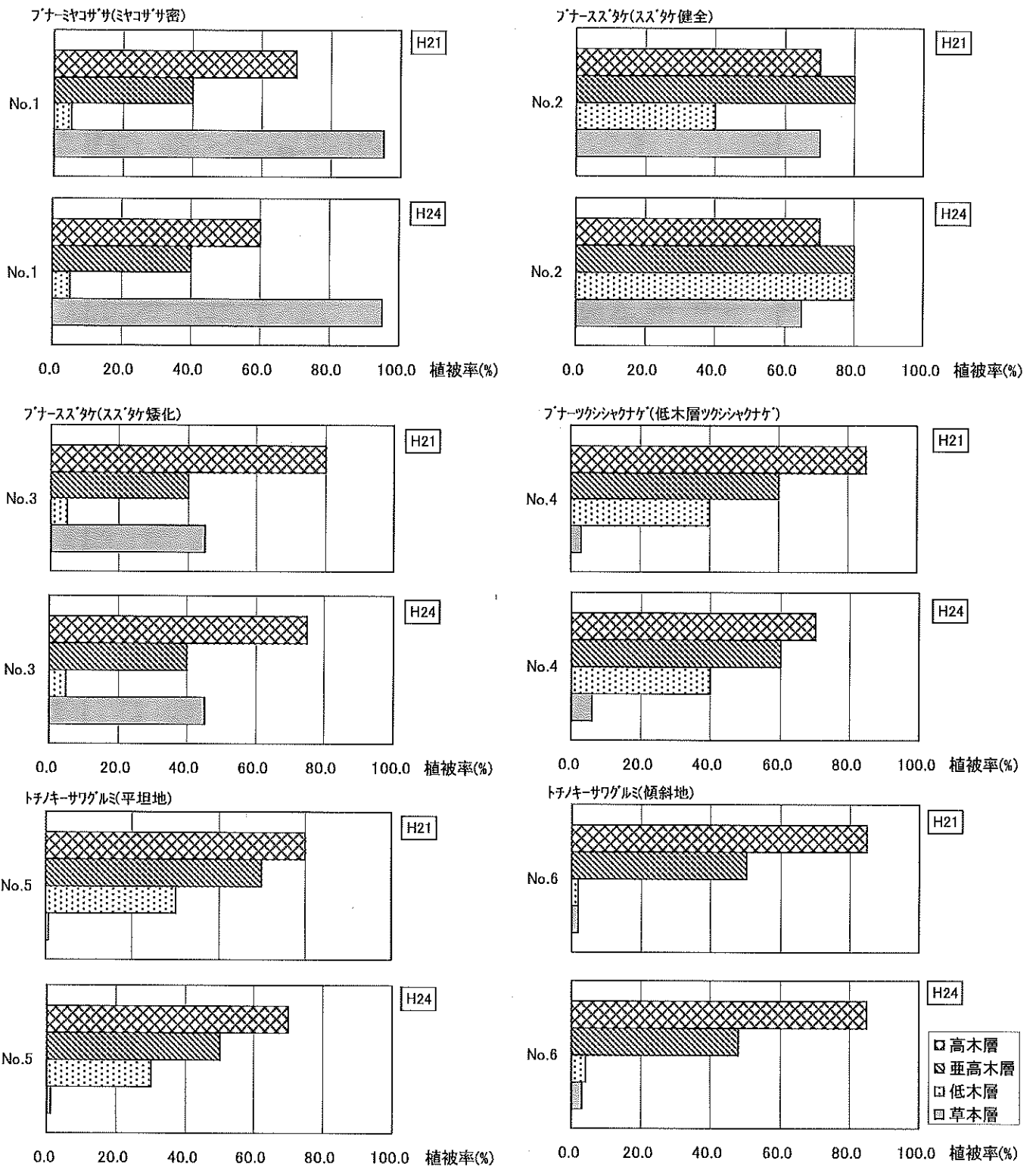
図 15 平成 21 (2009) 年度と 24 年度の各階層の植被率の変化
