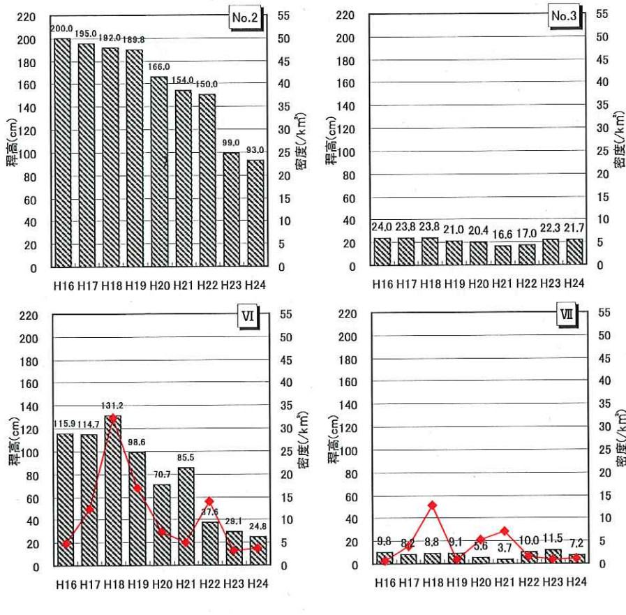
図 20(2) ササ型植生における平成 16～24 年度のズタケの稈高とニホンジカ生息密度の変化
