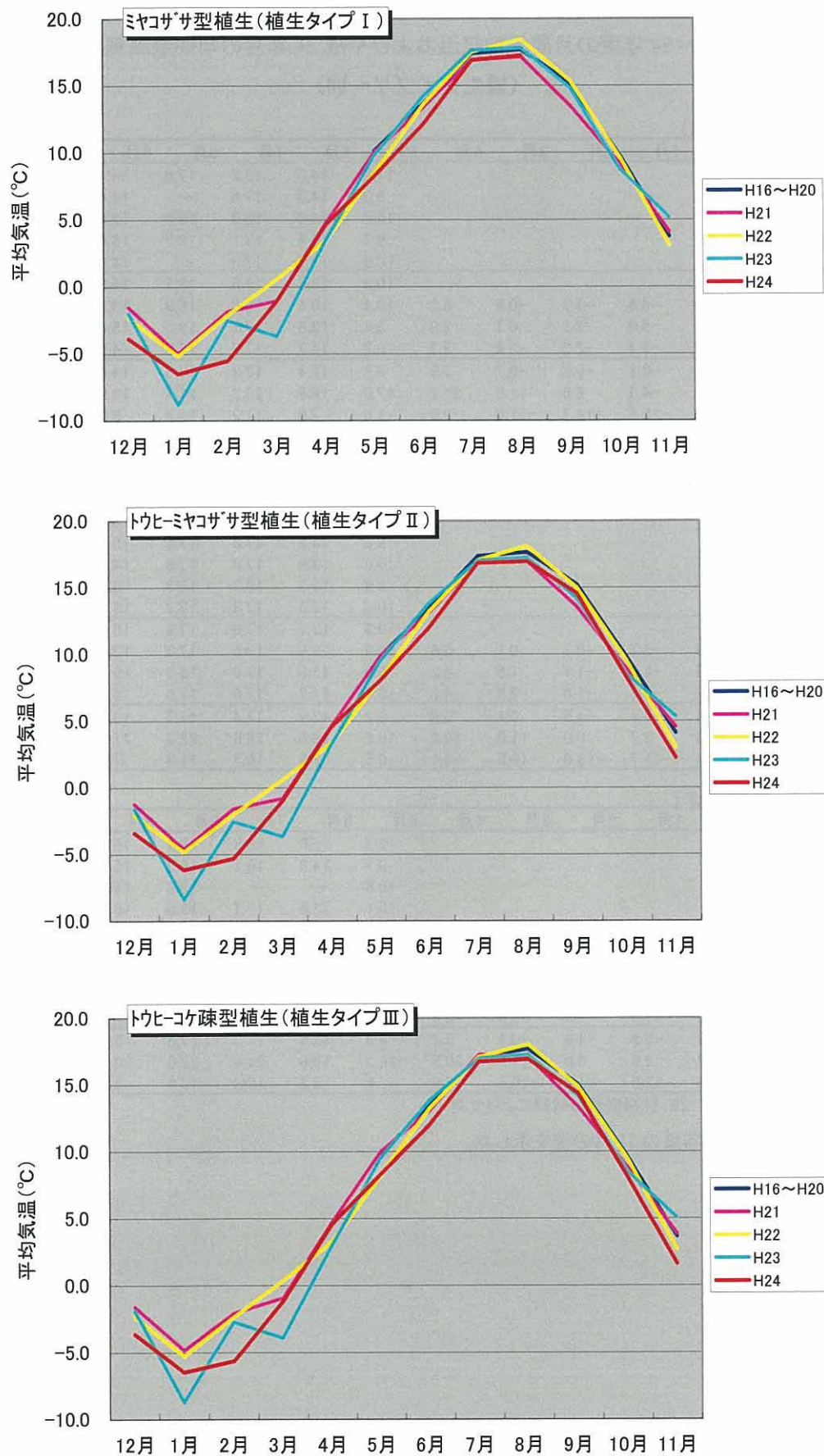
図 2(1) 平成 16~20 年度の 5 年間の月間平均気温の平均値と平成 21~24 年度の月間平均気温 (植生タイプⅠ~Ⅲ)
