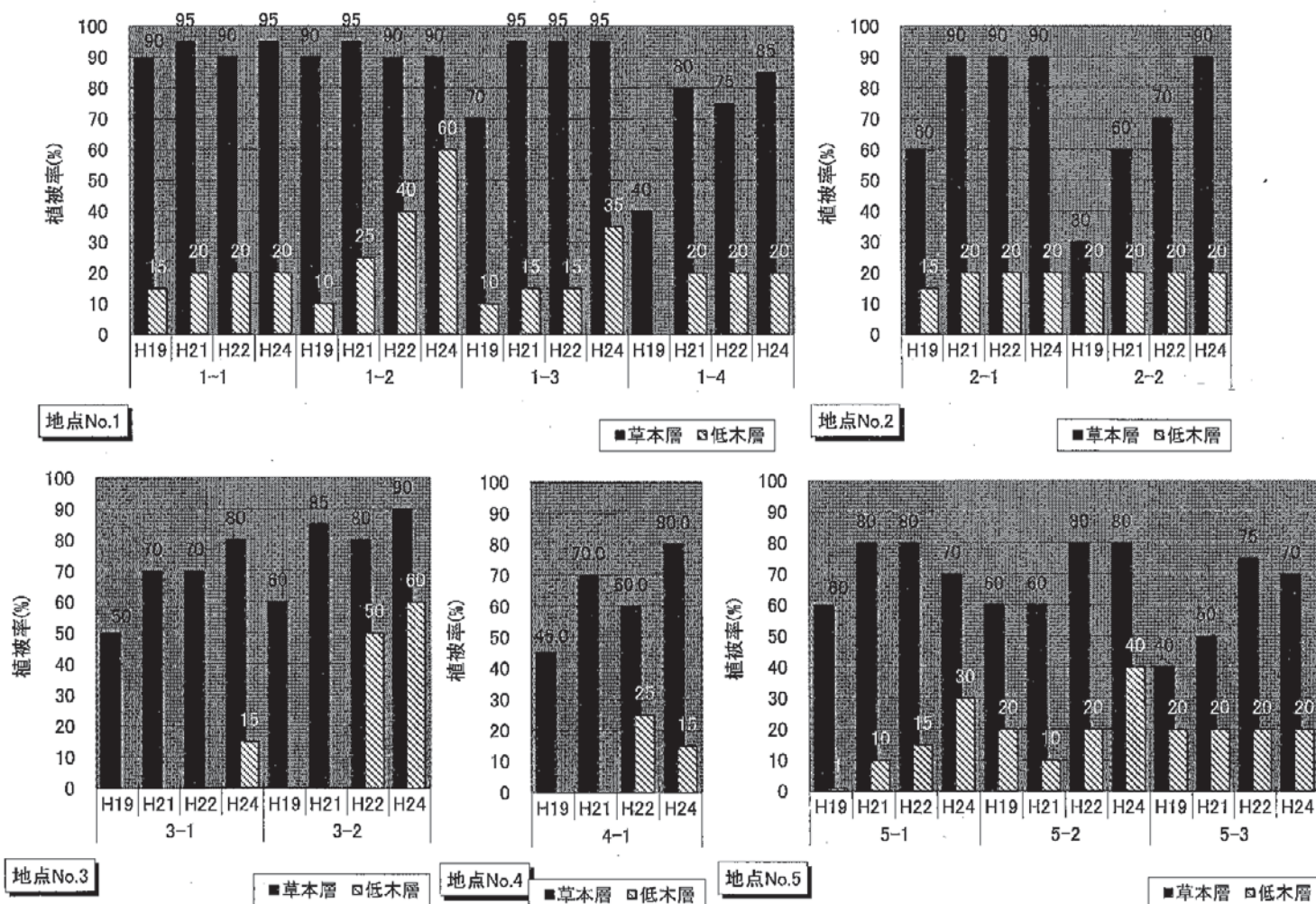
図 10 小規模防鹿柵内の草本層と低木層の植被率の変化
