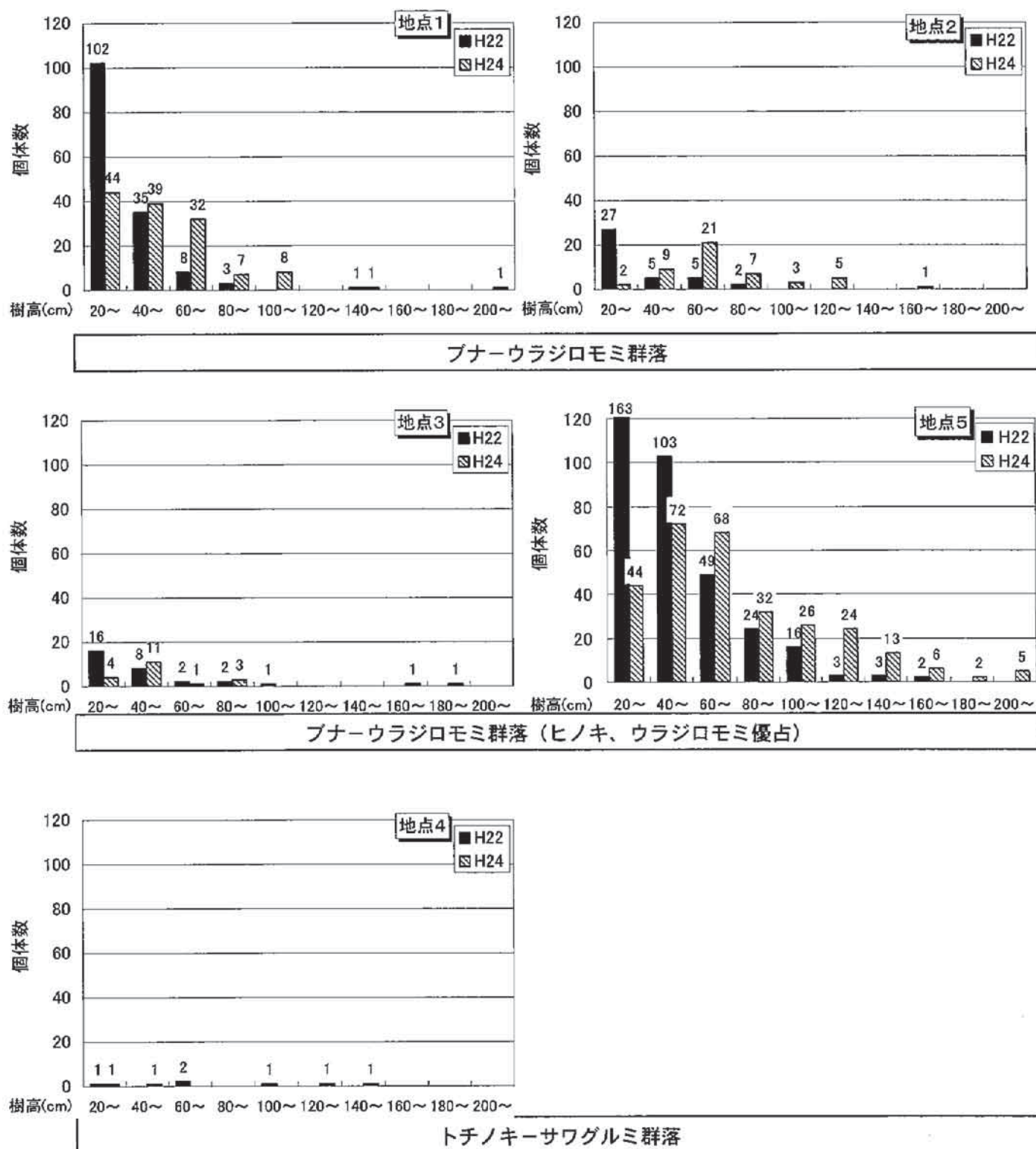
図 9(1) 平成 22 年度および平成 24 年度調査で確認された林冠構成種稚樹の樹高階級別個体数 (広葉樹)
