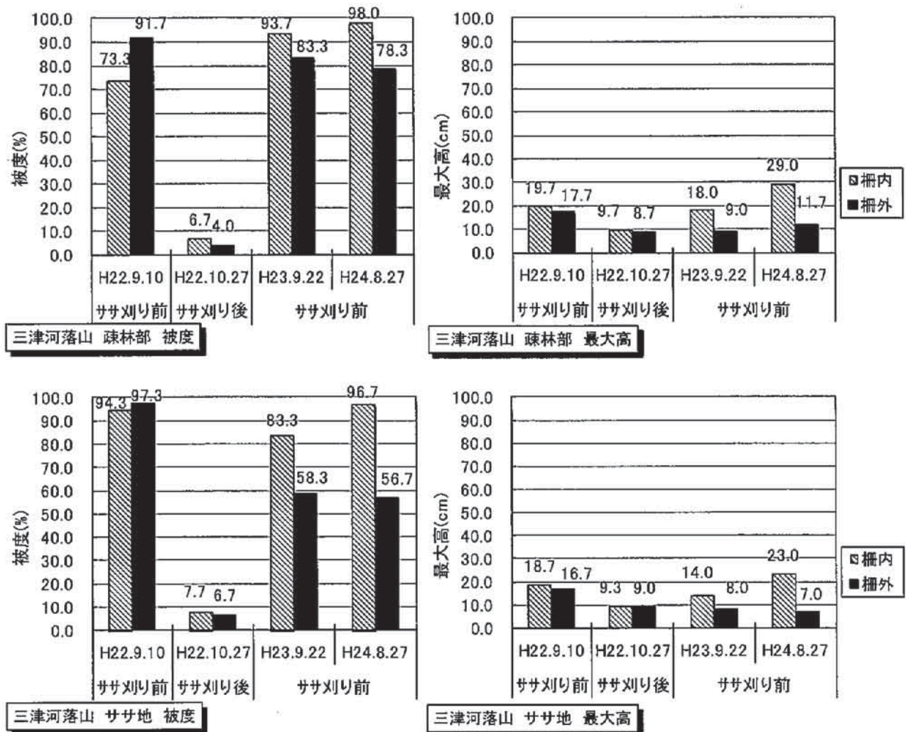
図 12 (2) 各植生調査区におけるササ刈り後のミヤコザサの被度および稈高の変化 (三津河落山試験区)
