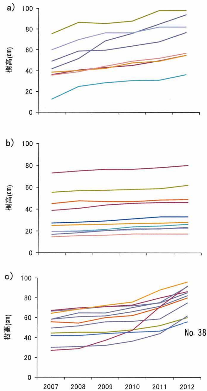
図 25 継続してササ刈りを行ったトウヒ稚樹の樹高の年変化
