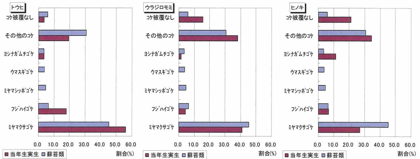
図 19 当年生実生が生育していた蘚苔類の種別割合と、倒木、根株上の蘚苔類の被覆率の関係
