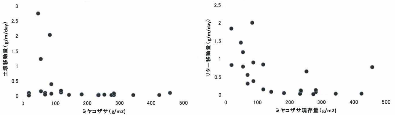
図 17 土壌とリターの移動量とミヤコザサ現存量との関係
