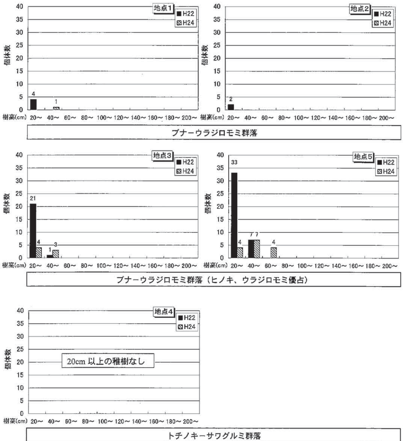
図 9(2) 平成 22 年度および平成 24 年度調査で確認された林冠構成種稚樹の樹高階級別個体数 (針葉樹)
