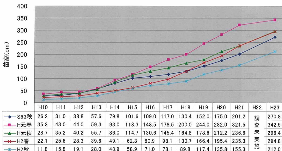
図 21 モニター木の播種時期別の平均苗高の変化（平成 10～23 年度）
