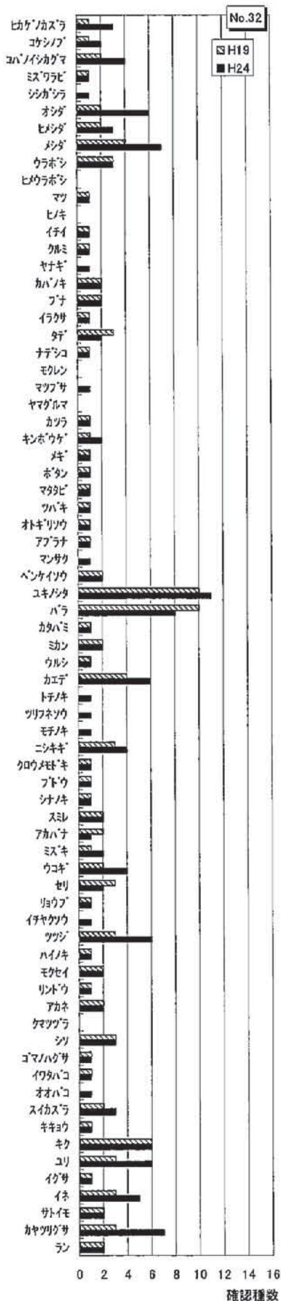
図7 科別確認種数の変化
