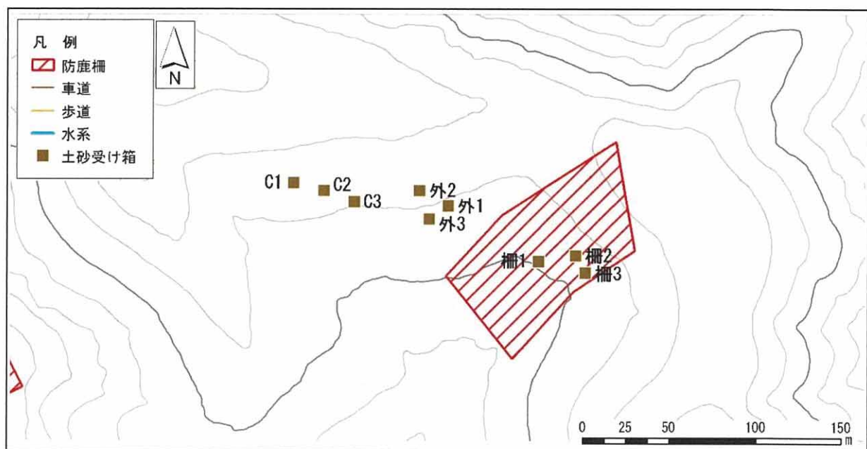
図 13(2) 土壌流出モニタリング地点（三津河落山試験区）
