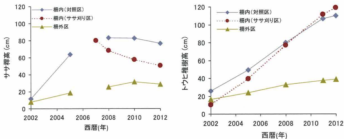
図 24 ササ稈高とトウヒ稚樹の年次変化
