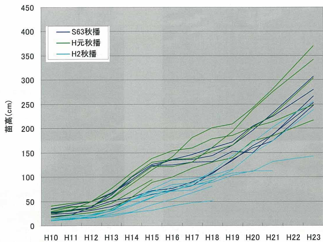
図 22 モニター木の個別成長曲線（平成 10～23 年度）
