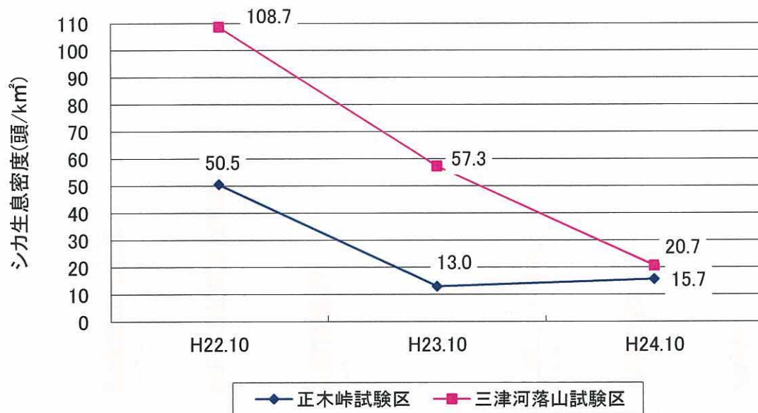
図 18 大規模ササ刈り区周辺部のニホンジカの生息密度の変化（平成 22～24 年度）
