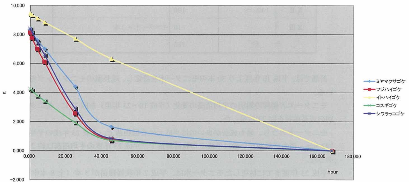
図 20 トウヒーミヤコザサ型植生における代表的な蘚苔類の時間経過に伴う含水量の変化
